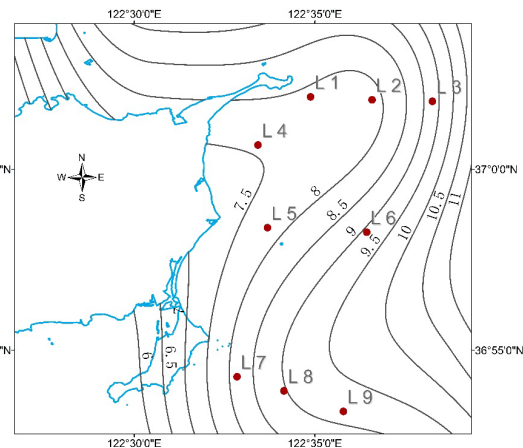
冬季小潮涨憩平均温度水平分布图
